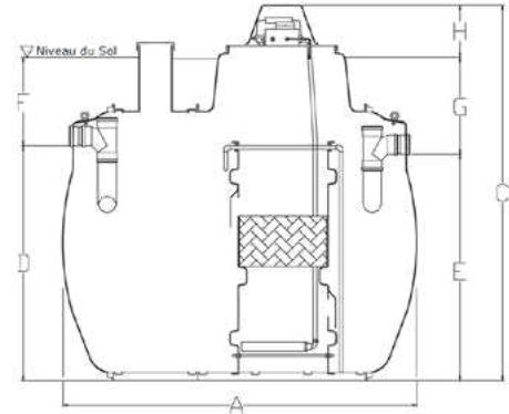
Tricel Novo avec pompe intégrée
